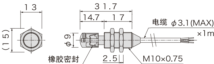
尺寸图
